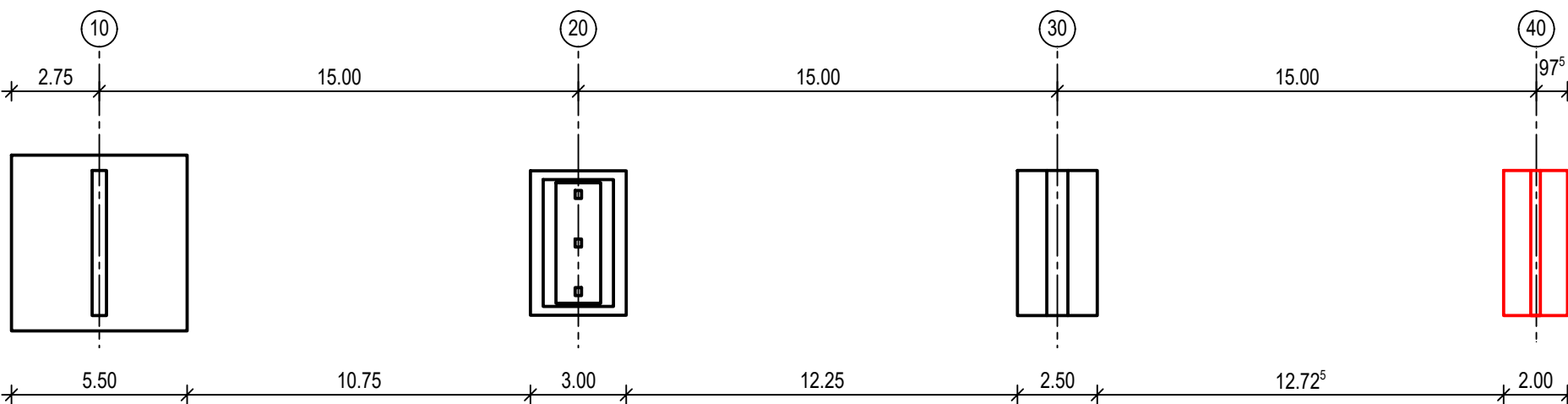
Übersicht 3-Feld-Brücke M1:200
